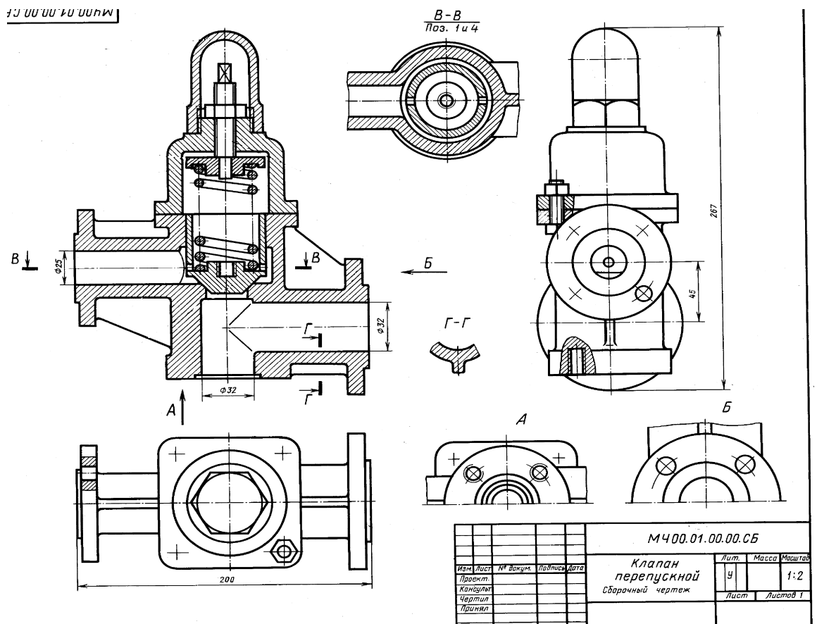
Сборочный чертеж изделия «Клапан перепускной»
